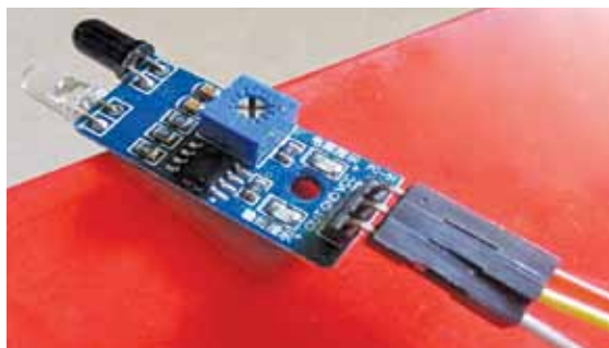
Fig. 3: IR sensor module
